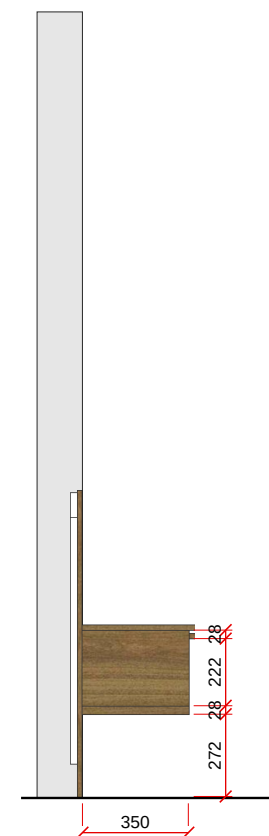
VISTA F - LATERAL - ESC. 1:25
