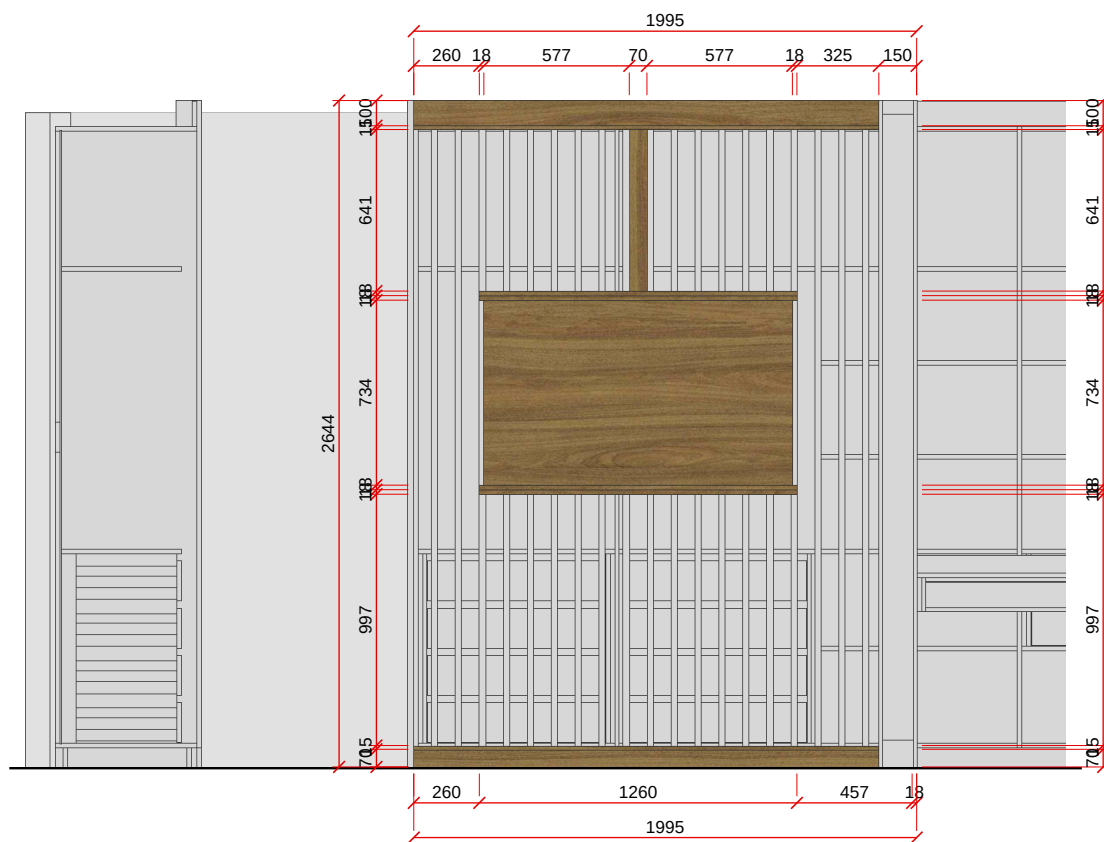
VISTA C - ESC. 1:30
