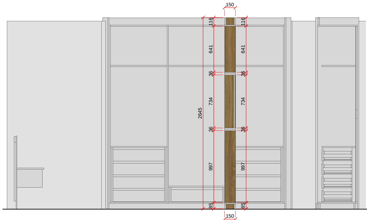
VISTA E - ESC. 1:30
