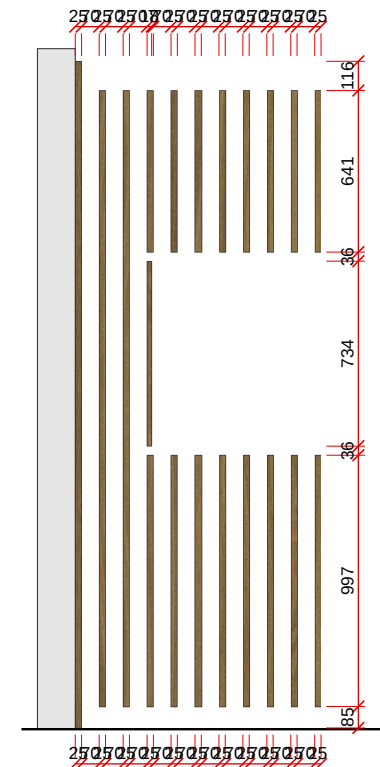
VISTA E - LATERAL - ESC. 1:30
