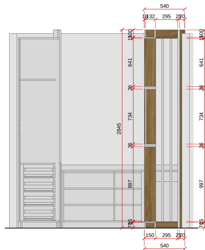
VISTA D - ESC. 1:30
